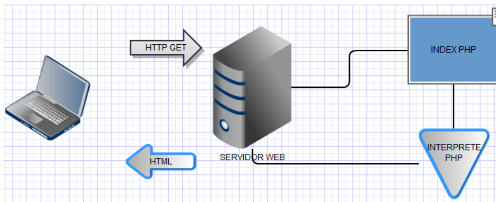
Figura 1. Ejecución PHP
